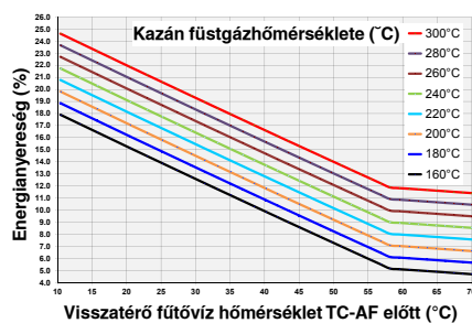
Energiamegtakarítás (a fűtővíz a ThermoCondensor aluFer®-be történő belépési hőmérsékletétől függően)
