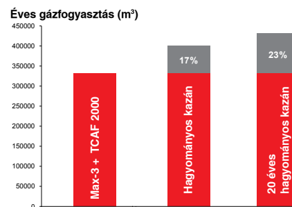
Éves gázmegetkarítás ThermoCondensor aluFer®-rel felszerelt kazánal összehasonlítva
